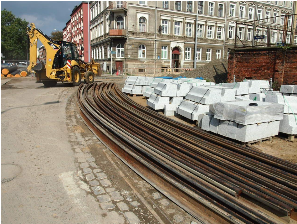
ul. Narutowicza – gięcie szyn nawierzchni torowej
