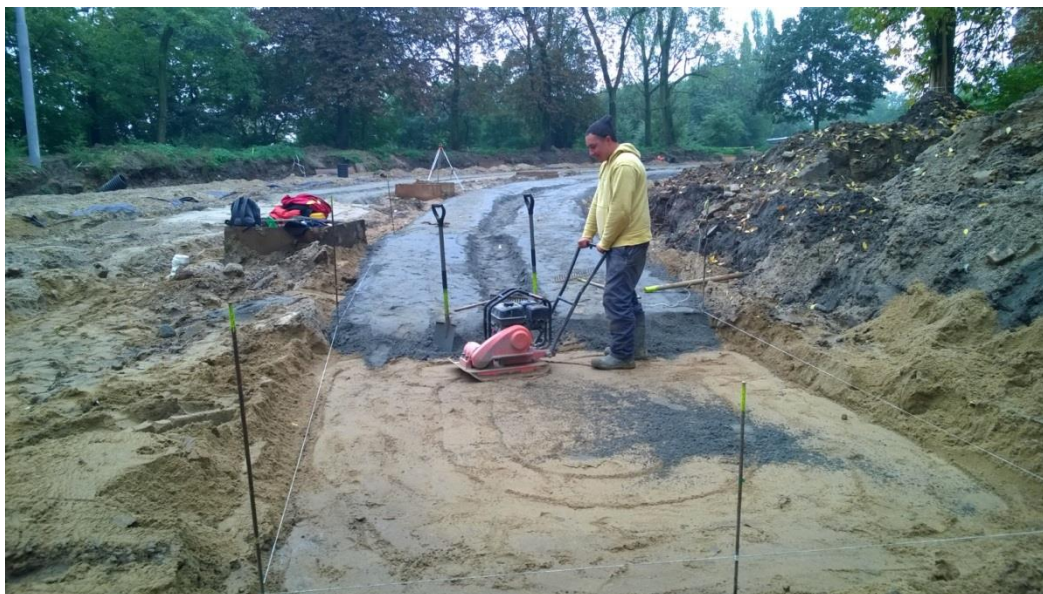
ul. Potulicka –wzmocnienie podłoża konstrukcji torowiska na pętli tramwajowej
